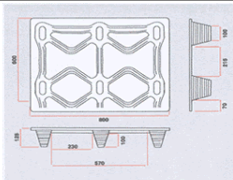
F 64 Belastning: 500 kg. Egenvekt 4,5 kg
