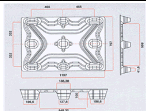
F 8 LF Belastning: 900 kg. Egenvekt 9 kg.
